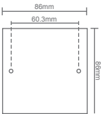
Dimensions BS 60669
